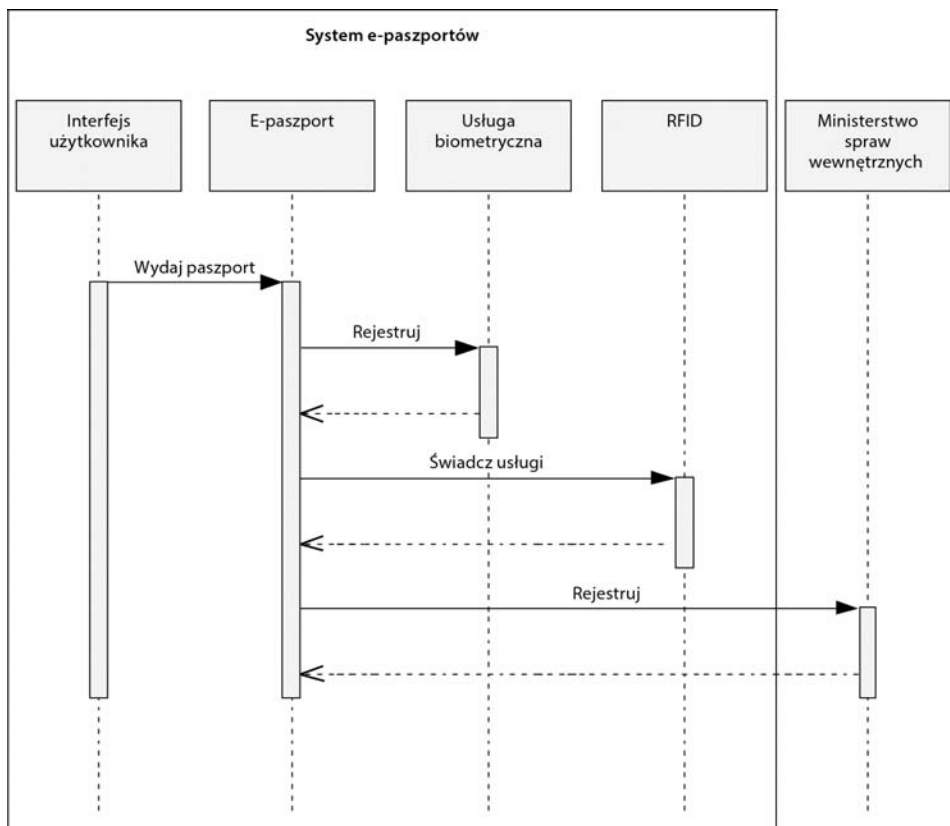
Rysunek 5.4. Proces rejestracji. Kiedy interfejs użytkownika (UI) wysyła do usługi e-paszportu zapytanie o wydanie paszportu, usługa, aby spełnić to żądanie, musi współpracować z kilkoma innymi usługami
