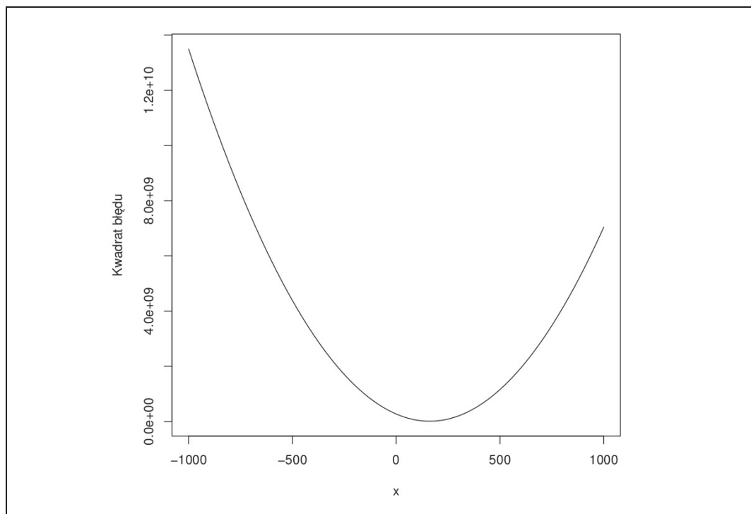
Rysunek 7.1. kwadrat błędu dla różnych wartości a
