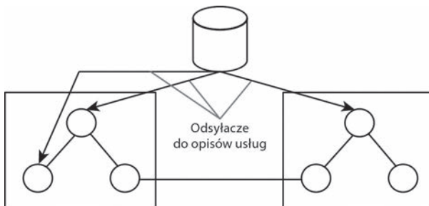
Rysunek 3.7. Rejestr jako mechanizm umożliwiający wykrywanie usług
