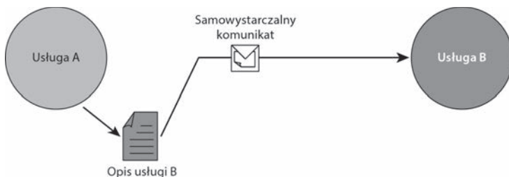
Rysunek 3.3. Komunikat istniejący jako niezależna jednostka komunikacji
