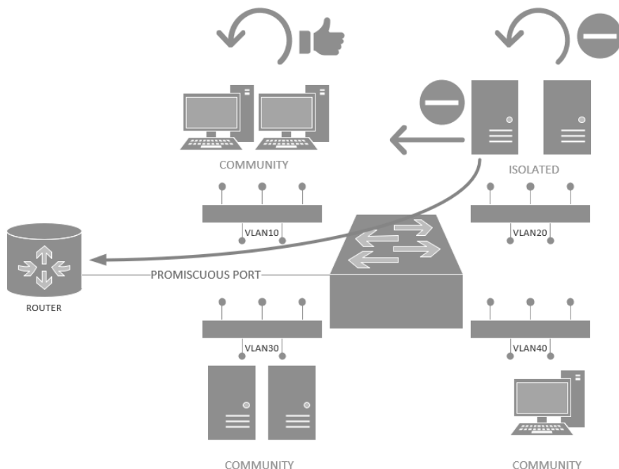
RYSUNEK 1.19. Komunikacja z sieci VLAN do routera dla PVLAN-u
