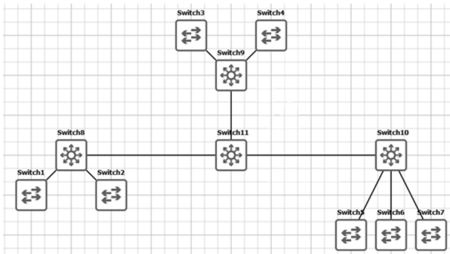
RYСУNEK 1.9. Warstwa rdzenia, dystrybucji oraz dostępu
