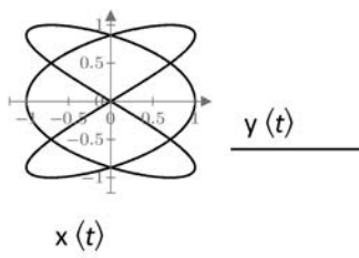
Rysunek 8.8. Wykres krzywej Lissajous w programie Mathcad PRIME, uzyskany dla a = 3 , b = 2 i \alpha = 0
