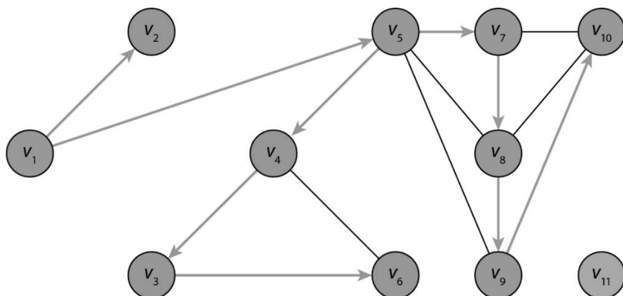
Rysunek 9.4. Trzeci krok algorytmu przeszukiwania w głąb
