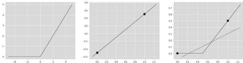
Rysunek 7.6: Wykres funkcji ReLU oraz jej zastosowanie do klasyfikacji nieliniowo separowalnych danych przedstawionych na środkowym rysunku. Po prawej stronie widoczne są dane po transformacji liniowej z dodaniem aktywacji sigmoidalnej, które można rozdzielić prawidłowo za pomocą linii.
