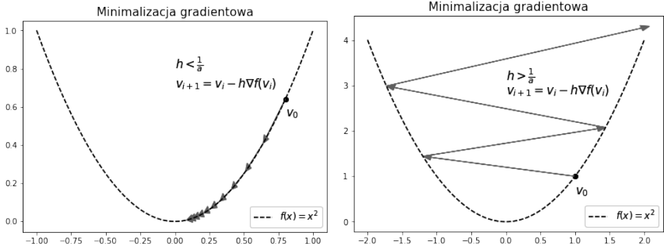
Rysunek 2.4: Wizualizacja minimalizacji gradientowej w zależności od wielkości kroku uczonego h .
