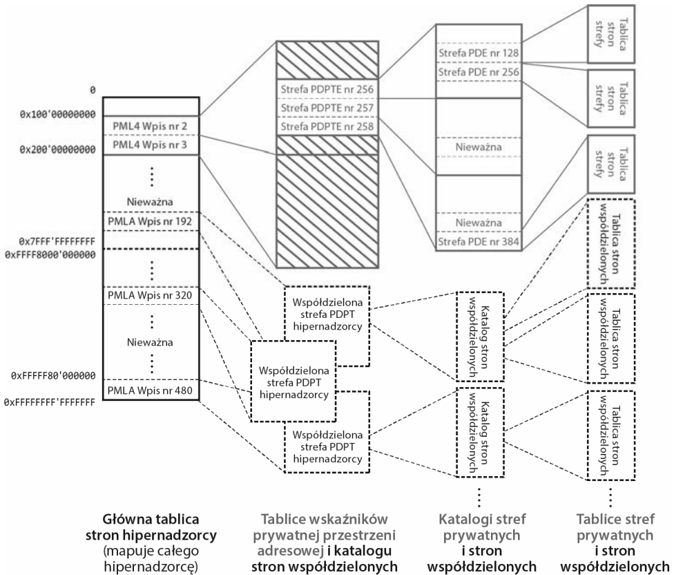
RYSUNEK 9.10. Prywatne przestrzenie adresowe hipernadzorcy i prywatne strefy pamięci
