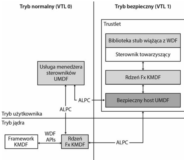
RYSUNEK 9.39. Architektura bezpiecznego towarzysza sterownika WDF
