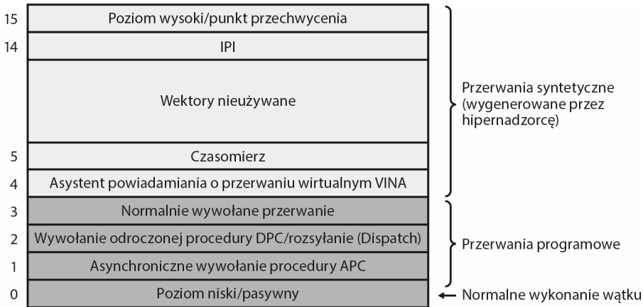
RYSUNEK 9.32. Poziomy żądania przerwań bezpiecznego jądra (IRQL)
