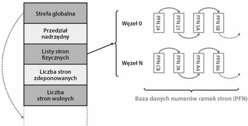
RYСУNEK 9.7. Przedział pamięci hipernadzorcy. Wirtualna przestrzeń adresowa dla strefy globalnej jest rezerwowana od końca struktury danych przedziału
