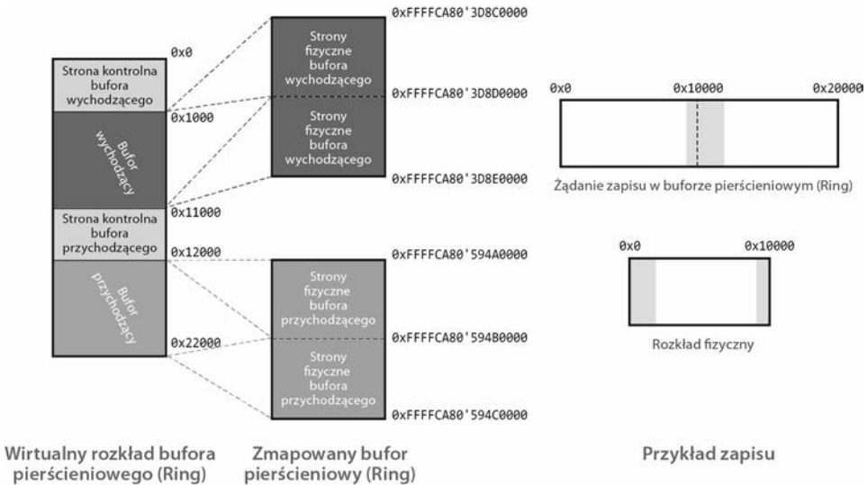
RYСУNEK 9.26. Przykład 16-stronicowego bufora pierścieniowego przydzielonego w partycji podrzędnej
