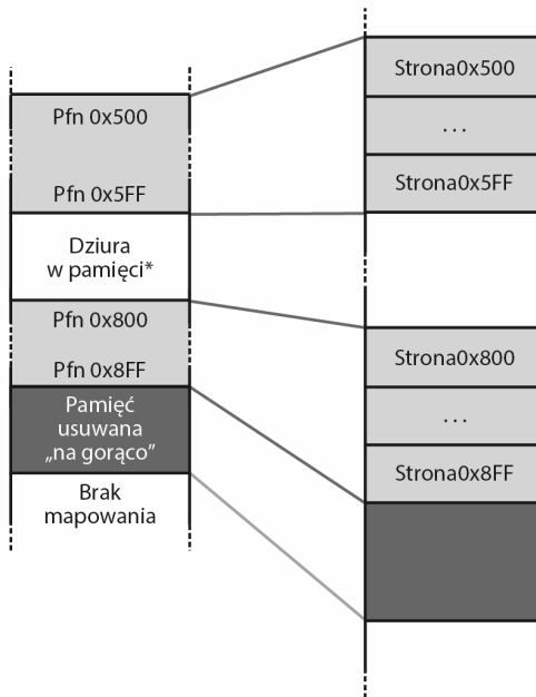
RYSUNEK 9.11. Przykład bazy danych PFN, w której usunięto część pamięci fizycznej
