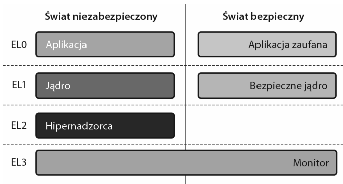
RYSUNEK 9.22. Środowisko wykonawcze procesora ARM64
