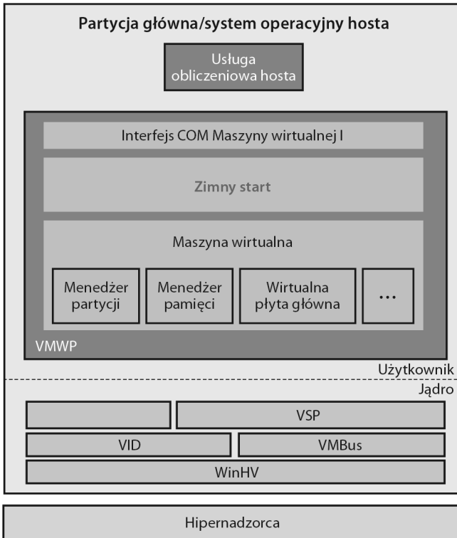
RYСУNEK 9.24. Proces roboczy maszyny wirtualnej i jego interfejs umożliwiający wykonanie „zimnego startu” maszyny wirtualnej
