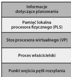
RYSUNEK 9.4. Struktura danych wątku hipernadzorcy
