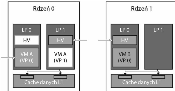
RYСУNEK 9.9. Łagodzenie skutków typu Hyperclear
