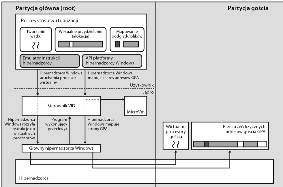
RYSUNEK 9.19. Architektura API platformy hipernadzorca Windows
