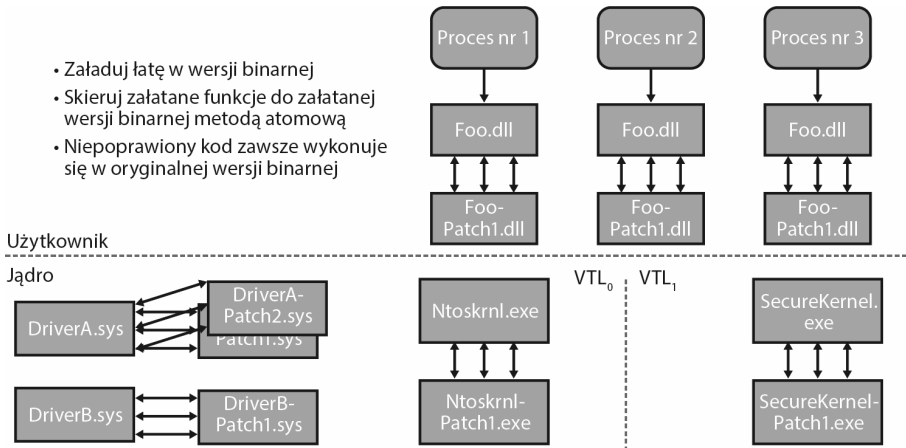
RYSUNEK 9.38. Schemat działania silnika do ładowania „na gorąco” na różnych typach binariów
