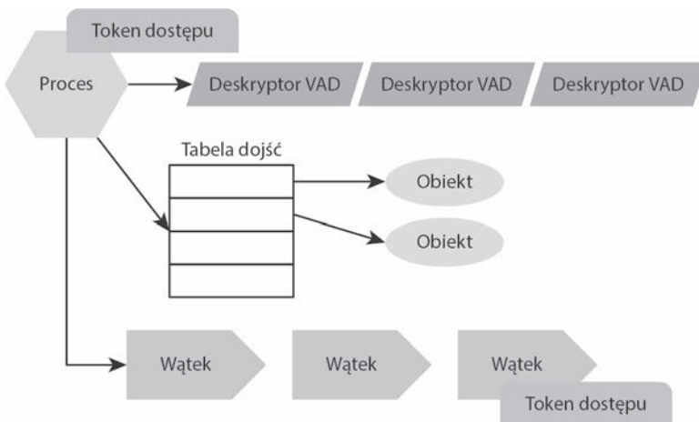
RYSUNEK 1.2. Proces i jego zasoby
