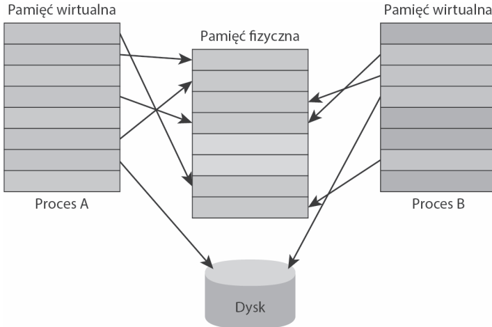
RYСУNEK 1.3. Mapowanie pamięci wirtualnej na pamięć fizyczną z zastosowaniem stronicowania
