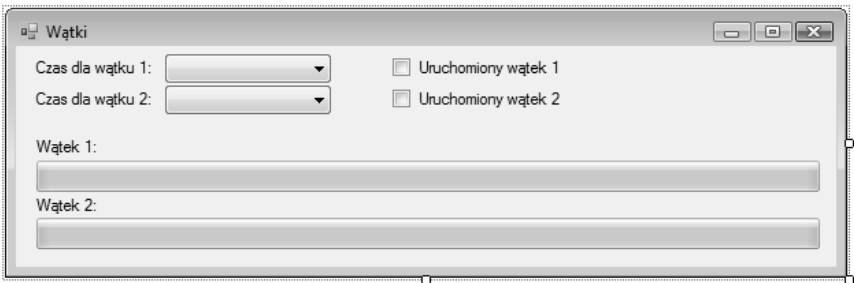
Rysunek 7.1. Rozmieszczenie komponentów w oknie głównym programu
