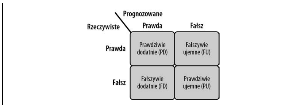
Rysunek 6.3. Binarna macierz pomyłek
