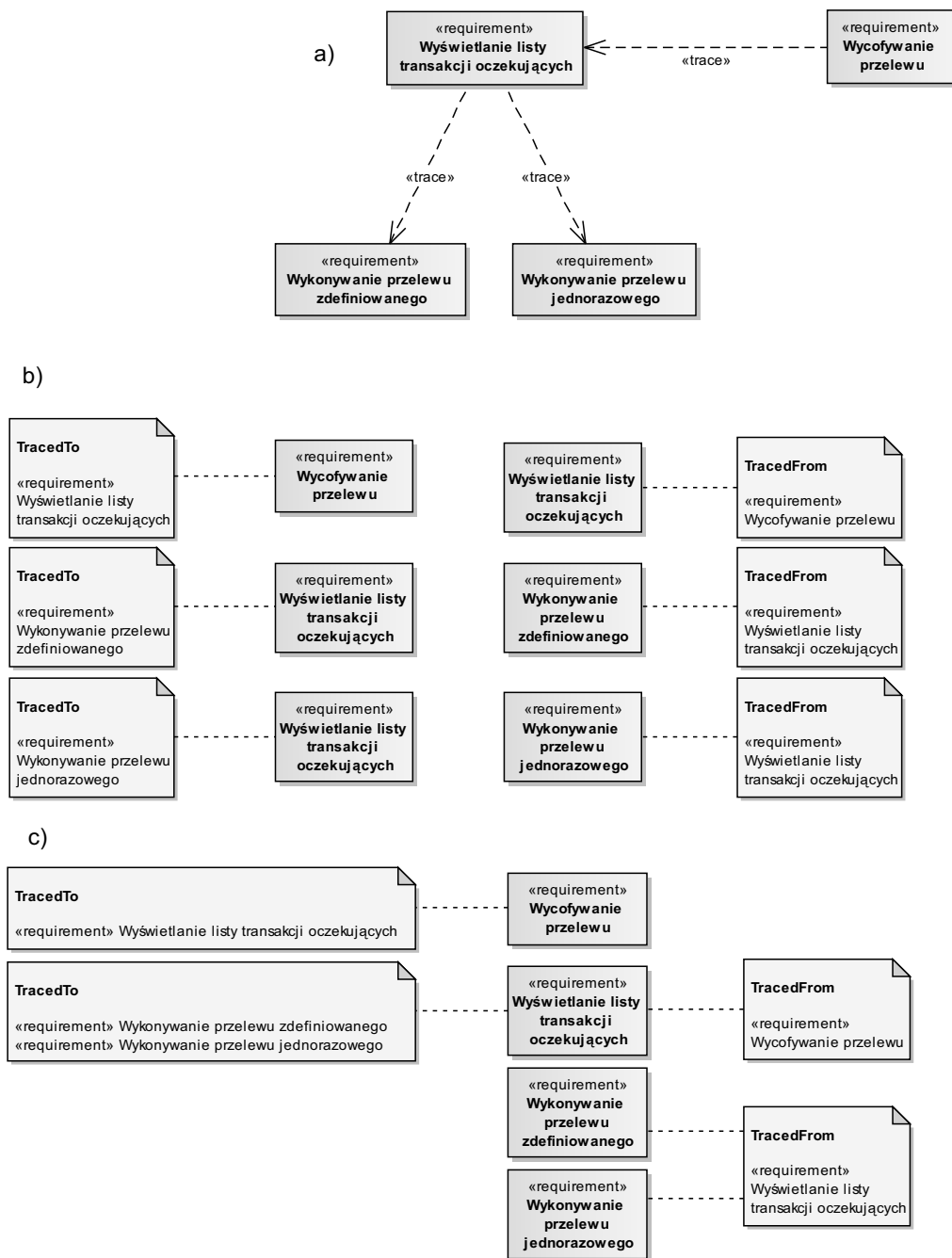
Rysunek 2.14. Różne konwencje graficznej prezentacji zależności śledzenia
