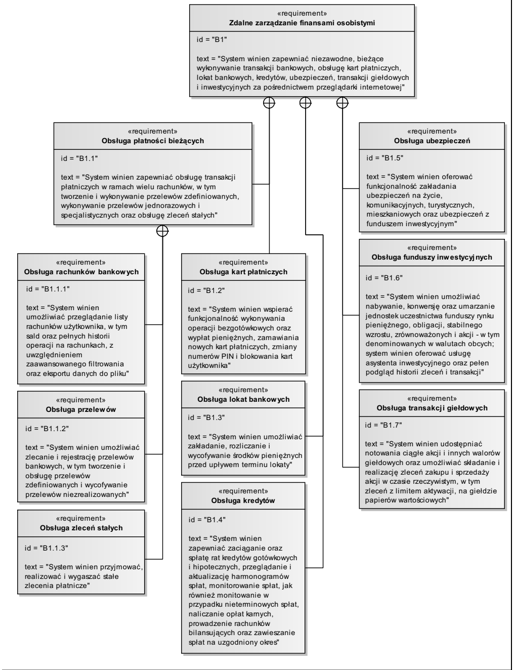
Rysunek 2.6. Wymagania funkcjonalne internetowej platformy transakcyjnej banku
