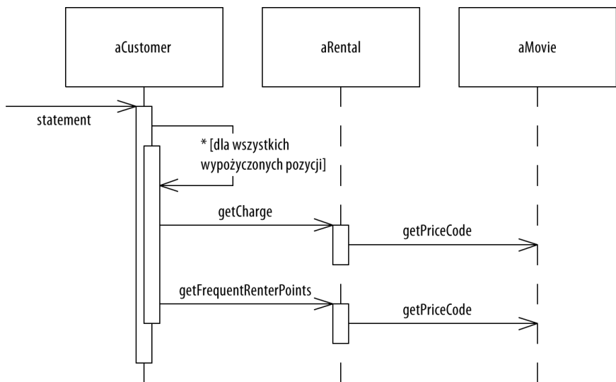
Rysunek 1.7. Diagram sekwencji po ekstrakcji i przeniesieniu obliczania punktów stałego klienta
