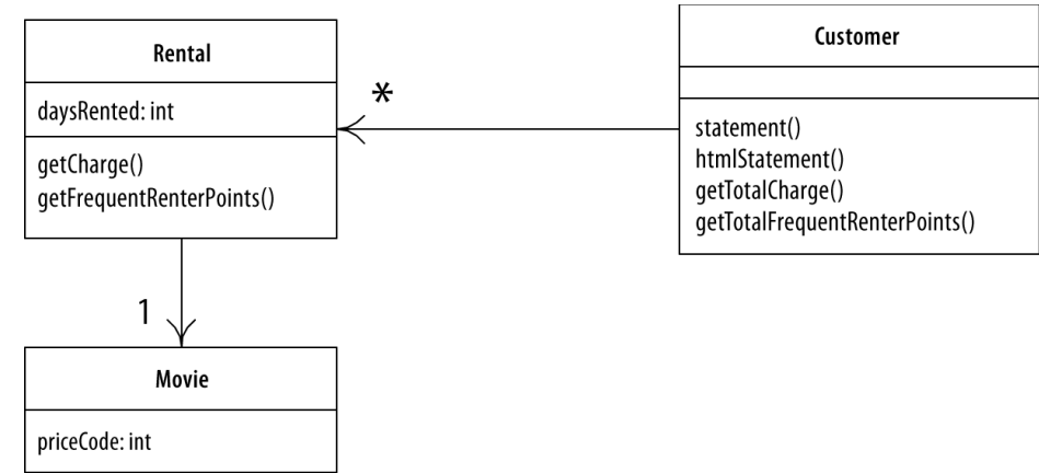
Rysunek 1.12. Diagram klas przed przeniesieniem metod do klasy Movie
