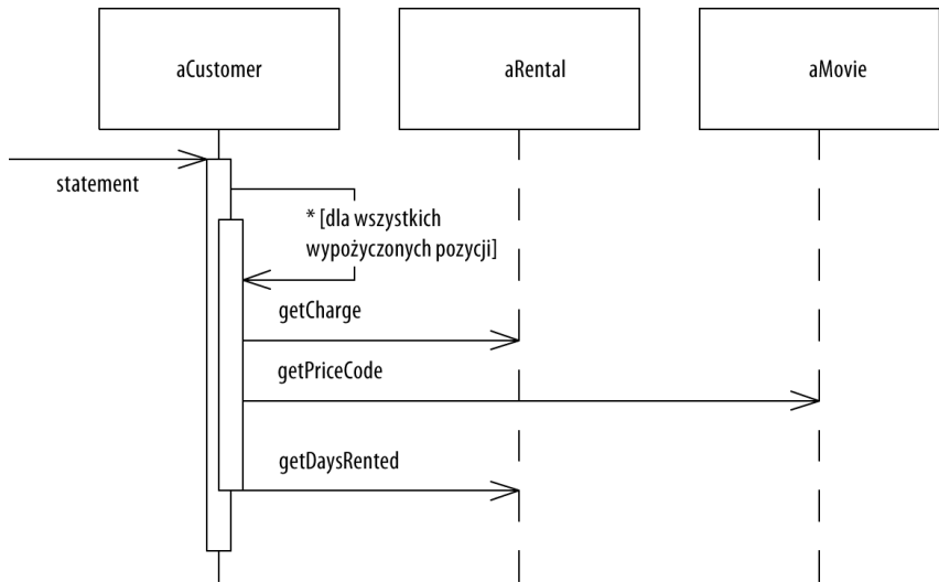
Rysunek 1.5. Diagram sekwencji przed ekstrakcją i przeniesieniem obliczania punktów stałego klienta
