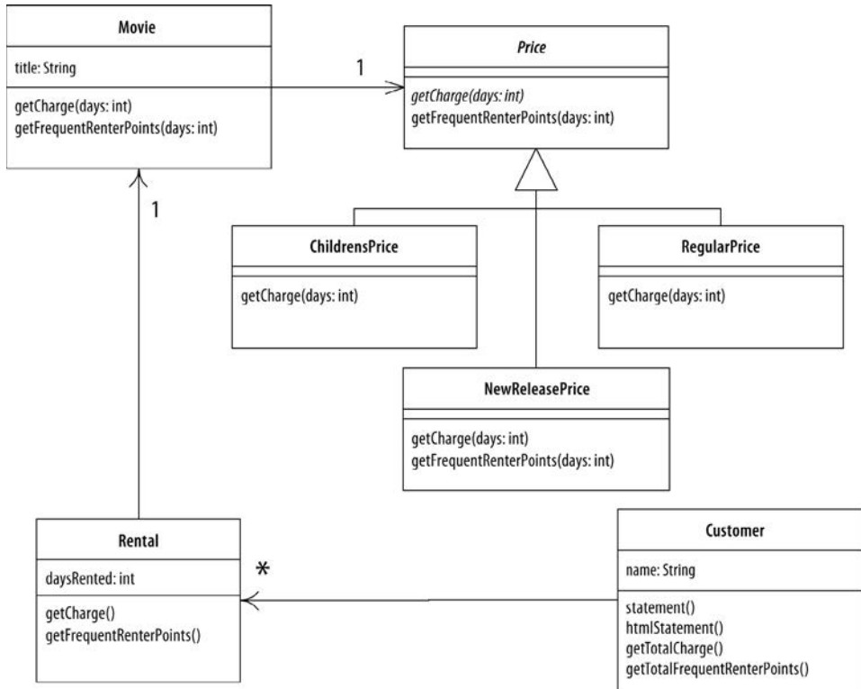
Rysunek 1.17. Diagram klas po zastosowaniu wzorca Stan
