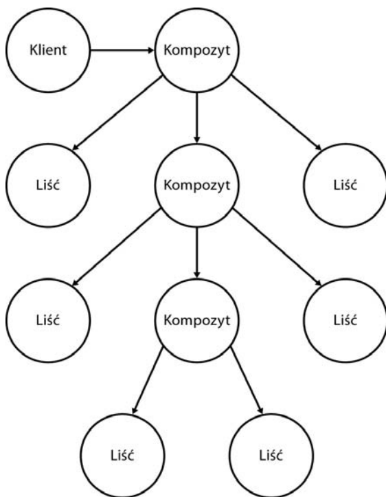
RYСУNEK 7.6. Graf ilustrujący strukturę działającej aplikacji
