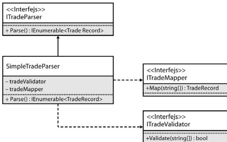
RYСУNEK 7.2. Klasa SimpleTradeParser również została podzielona na mniejsze klasy o pojedynczych odpowiedzialnościach
