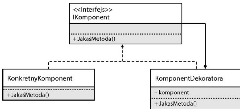
RYСУNEK 7.4. Diagram UML-a wzorca Dekorator
