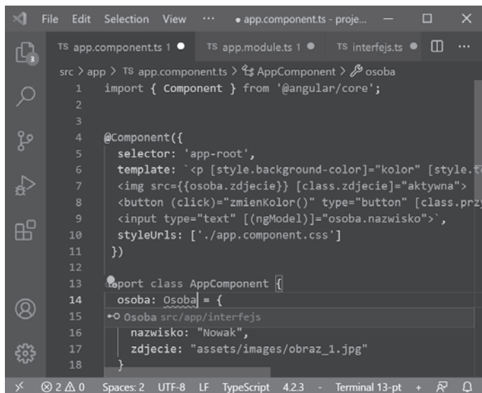
Rysunek 2.49. Użycie skrótu Ctrl+I
