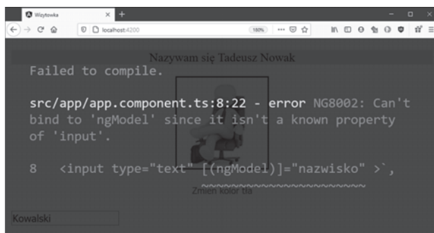
Rysunek 2.47. Błąd — nieznaną właściwość ngModel
