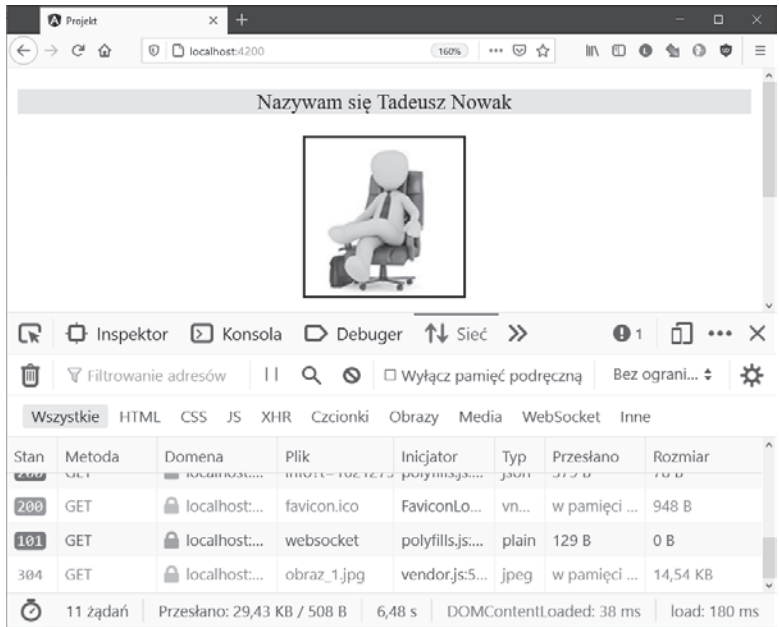
Rysunek 2.51. Spółdziałanie dyrektywy ngIf
