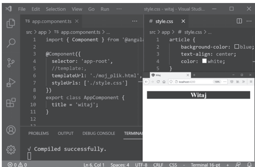
Rysunek 2.41. Definicja stylu CSS zapisanego we własnym pliku
