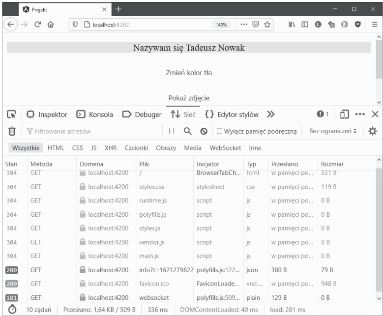
Rysunek 2.50. Spółdziałanie dyrektywy ngIf
