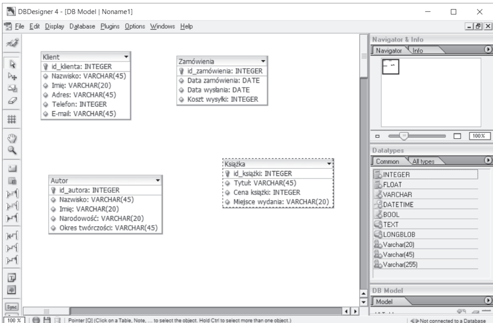
Rysunek 1.18. Tabele zaprojektowane w programie DBDesigner4
