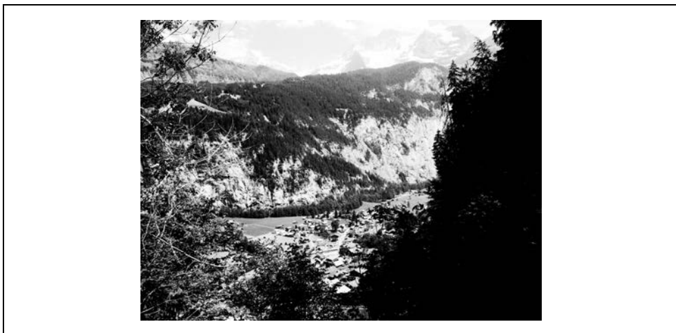
Rysunek 3.7. Szwajcarskie Alpy. Optymalizacja przypomina wędrówkę po wykresie funkcji. Miejscem docelowym jest dno najniższej doliny (minimalizacja) lub szczyt najwyższego wzniesienia (maksymalizacja). Potrzebujemy dwóch rzeczy: współrzędnych punktów minimalizacji lub maksymalizacji oraz wysokości wykresu w tych punktach
