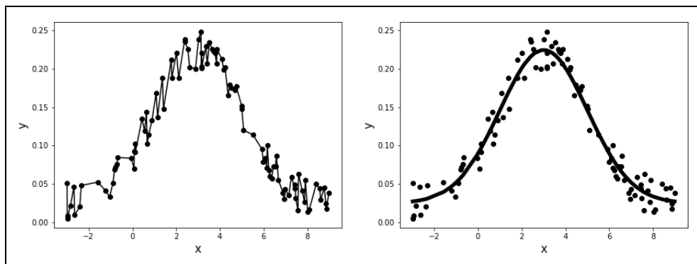
Rysunek 3.1. Po lewej: funkcja dopasowania idealnie pasuje do danych; nie jest to jednak dobra funkcja prognozowania, ponieważ dopasowuje szumy w danych zamiast głównego sygnału. Po prawej: bardziej regularna funkcja dopasowana do tego samego zbioru danych. Użycie tej funkcji zamiast funkcji z lewej części wykresu zapewni lepsze prognozy, nawet jeśli funkcja po lewej lepiej pasuje do punktów danych
