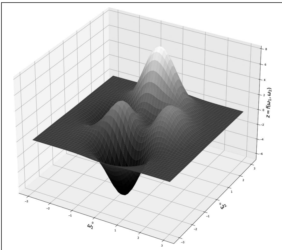
Rysunek 3.10. Wykres funkcji niewypukłej obejmuje szczyty, doliny i punkty siodłowe. Problem minimalizacji na takim wykresie wiąże się z ryzykiem utknięcia w minimach lokalnych i niezalezienia minimów globalnych
