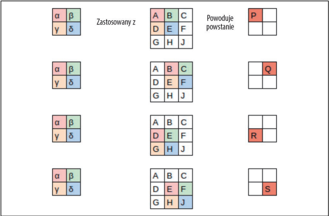
Rysunek 13.7. Stosowanie jądra splotu
