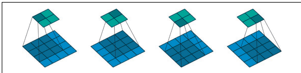
Rysunek 13.3. Wynik zastosowania jądra 3×3 w obrazie 4×4 (dzięki uprzejmości Vincenta Dumoulina i Francesco Visina)
