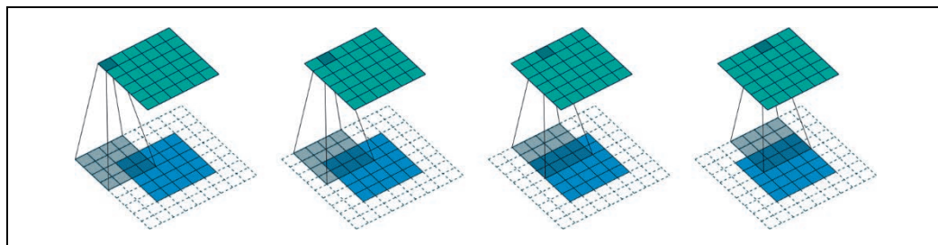
Rysunek 13.5. Jądro spłotu 4×4 używane z danymi wejściowymi o rozmiarze 5×5 i dwoma pikselami wypełnienia (dzięki uprzejmości Vincenta Dumoulina i Francesco Visina)
