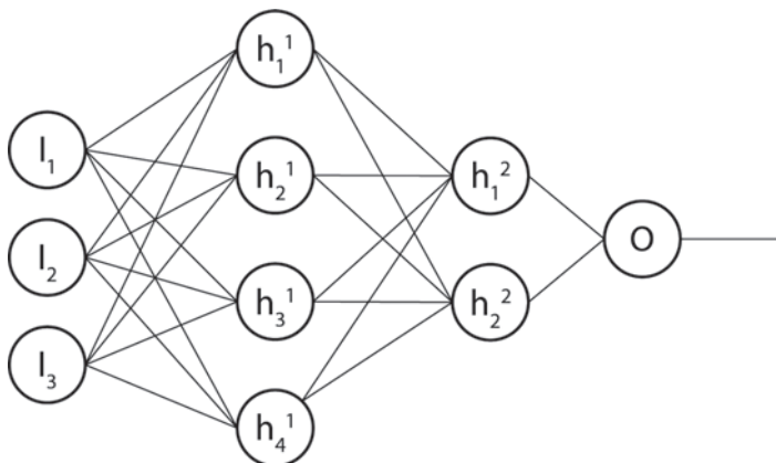
Rysunek 1.14. Perceptron wielowarstwow (MLP) z dwiema warstwami ukrytymi. Trzy węzły wejściowe są połączone z pierwszą warstwą ukrytą ( h^1 ), a warstwa h^1 jest połączona z drugą warstwą ukrytą ( h^2 ), która jest połączona z neuronem wyjściowym
