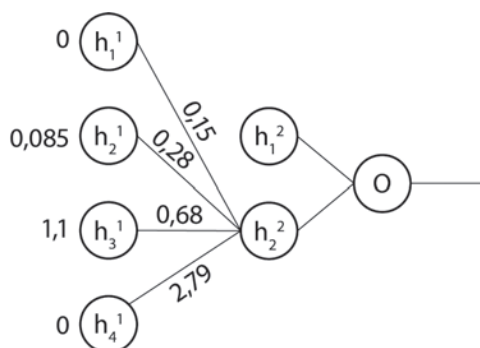
Rysunek 1.20. Wartości wejściowe i wagi połączeń z węzłem h_2^2
