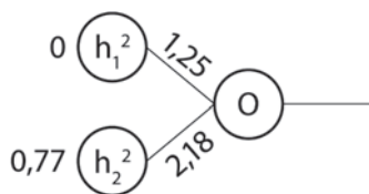
Rysunek 1.21. Wyjście warstwy h^2 jako wejście warstwy wyjściowej oraz wagi połączeń z warstwą wyjściową
