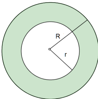
Rysunek 8: Pierścień kołowy
