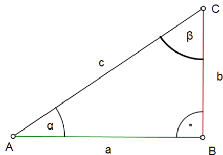
Rysunek 16: Bok b jest przyprostokątną wychodzącą z wierzchołka C kąta \beta , a bok a jest przyprostokątną leżącą naprzeciwko tego kąta. Stosunek długości boku a do długości boku b jest więc tangensem kąta \beta , który oznaczamy przez \operatorname{tg} \beta
