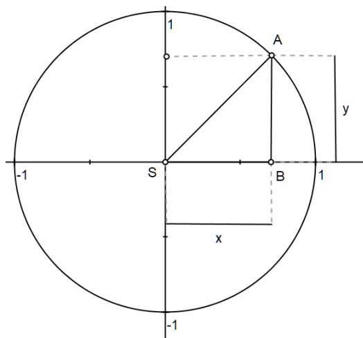
Rysunek 21: Długość boku SB jest równa współrzędnej x -owej punktu A , natomiast długość boku BA jest równa y -owej współrzędnej tego punktu
