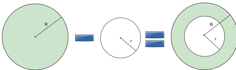
Rysunek 9: “Powstanie” pierścienia kołowego
