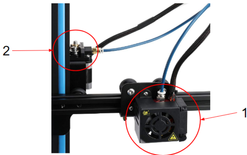
Zdj.2.1.3. Ekstruder typu Bowden, 1-ekstruder, 2-układ napędowy prowadzący filament do ekstrudera.
