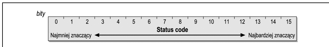
Rysunek 4.30. Pole Status Code
