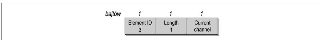
Rysunek 4.35. Element informacyjny DS Parameter Set
