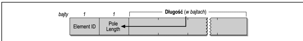
Rysunek 4.31. Element informacyjny ramki zarządzającej
