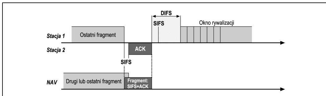
Rysunek 4.2. Ustawienia pola Duration w ostatnim fragmencie
