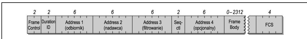
Rysunek 4.1. Generalny schemat ramki danych
