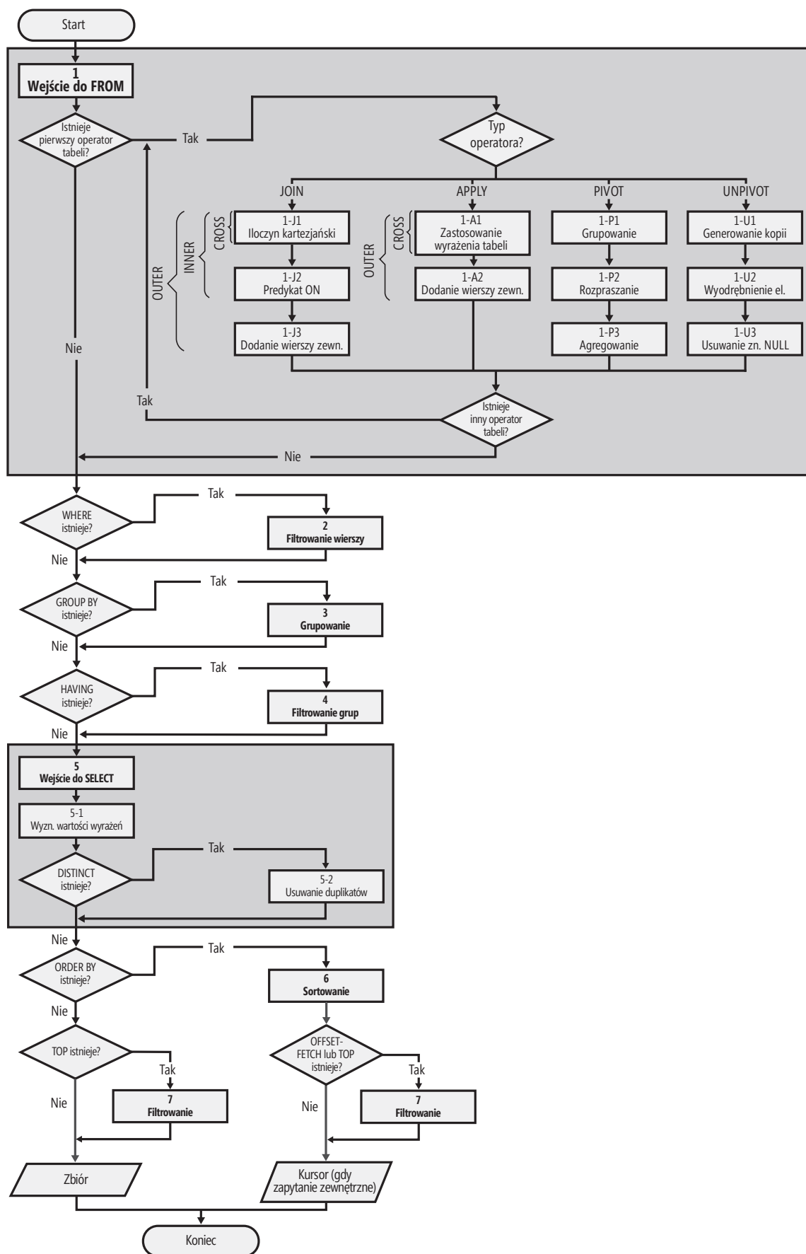
RYСУNEK 1-1 Diagram przepływu ilustrujący logiczne przetwarzanie zapytania.
