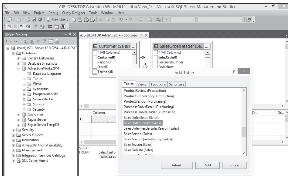
RYSUNEK 12.2. Widok przedstawiający złączenie ze sobą tabel Sales.Customer i Sales.SalesOrderHeader
