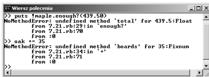
Rysunek 7.21. Różne rodzaje błędów, które mogą wystąpić, jeśli metody i operatory będą wywoływane z niewłaściwymi typami lub operandami
