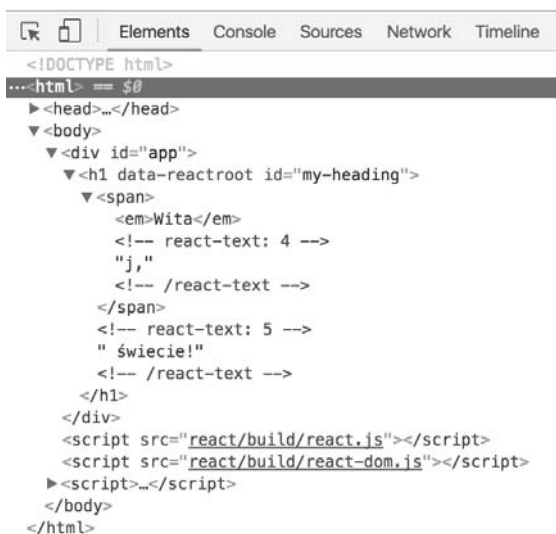
Rysunek 1.5. Kod HTML wygenerowany poprzez zagnieżdżone wywołania React.DOM
