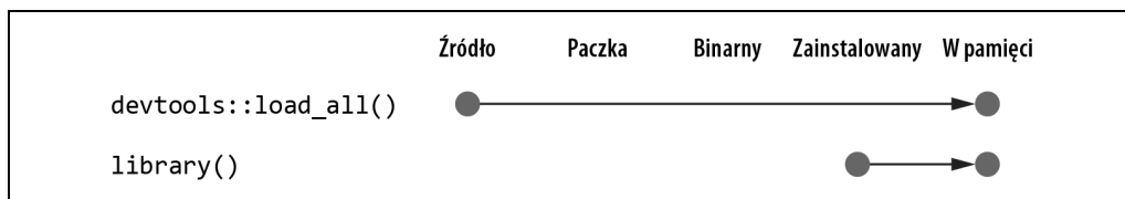
Rysunek 4.4. Wywołanie devtools::load_all() kontra library()
