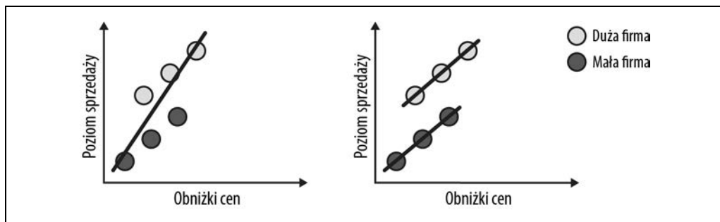
Rysunek 1.4. Błąd systematyczny a paradoks Simpsona
