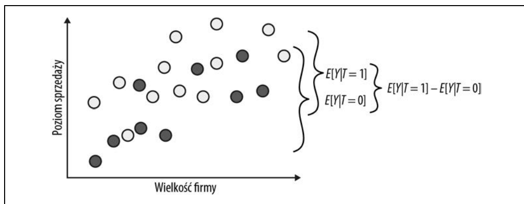
Rysunek 1.8. Wykres po usunięciu niezrealizowanych potencjalnych wyników
