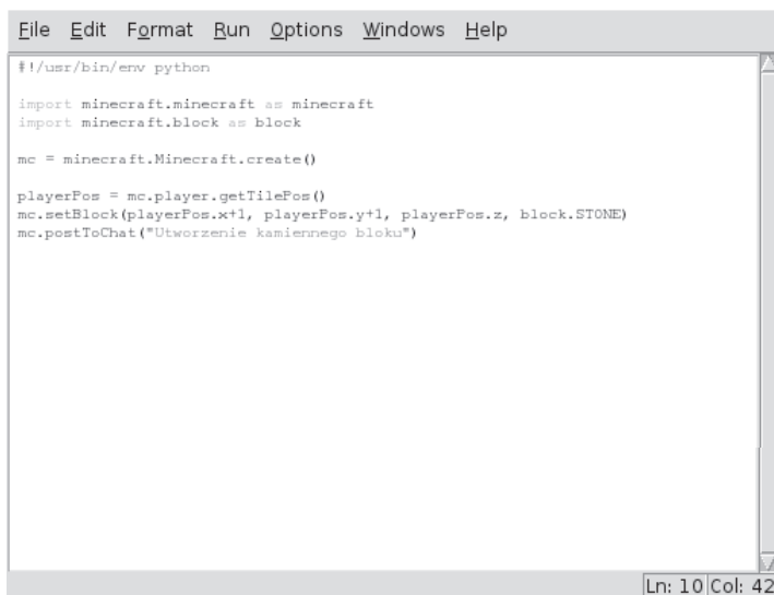
Rysunek 13.6. Gotowy program modyfikujący grę Minecraft Pi Edition
