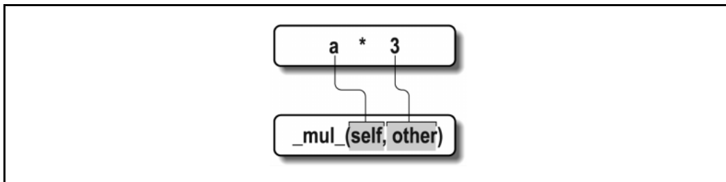
Rysunek 6.3. Odzwierciedlanie operatorów w metodach specjalnych
