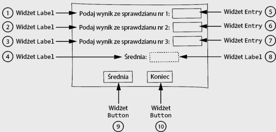
Rysunek 13.19. Szkic okna budowanego programu
