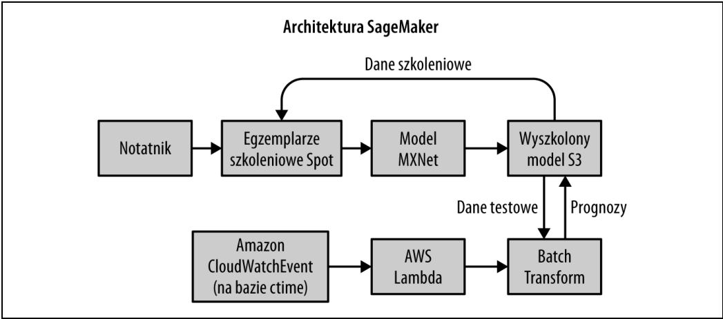
Rysunek 14.7. Amazon SageMaker
