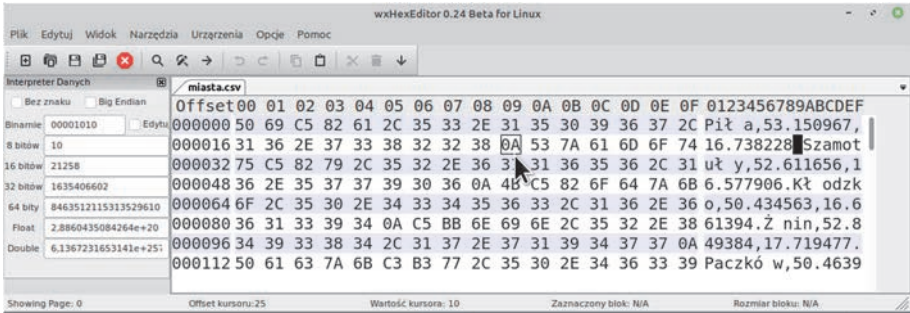
Rysunek 6.2. Plik z danymi wyświetlony w oknie edytora heksadecymalnego
