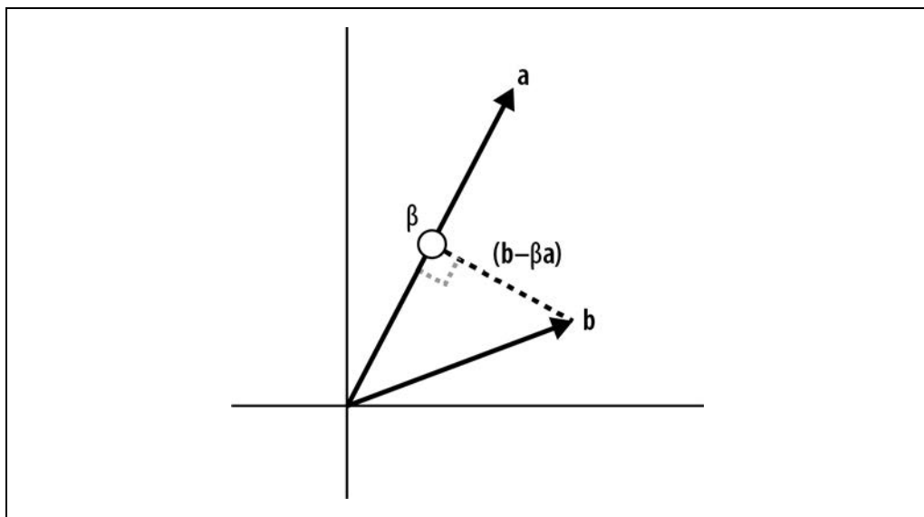
Rysunek 2.6. Do znalezienia rzutu punktu znajdującego się w końcu wektora b na wektor a minimalizującego odległość potrzebujemy wzoru na \beta , dla którego długość wektora \mathbf{b} - \beta\mathbf{a} jest możliwie najmniejsza
