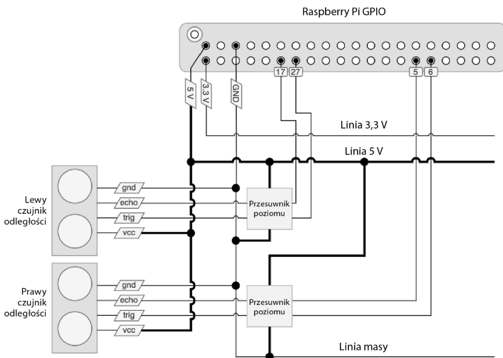
Rysunek 8.5. Podłączenie czujników HC-SR04 do przesuwników poziomu
