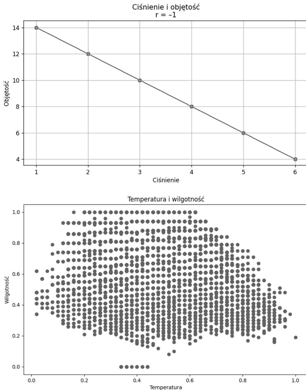
Rysunek 1.12. Zmienne skorelowane ujemnie
