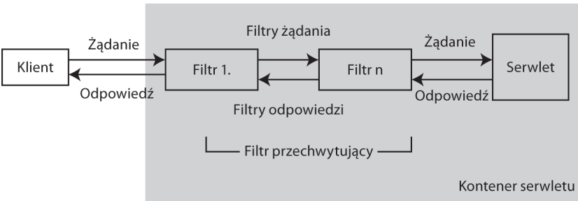
Rysunek 3.8. Wzorec Filtr Przechwytyjący
