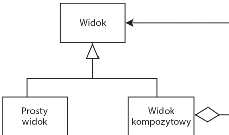
Rysunek 3.12. Diagram klas wzorca Widok Kompozytowy
