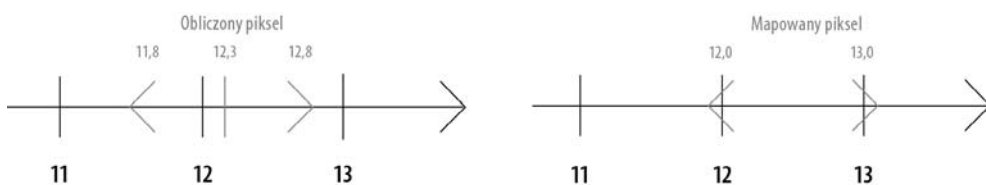
Rysunek 13.9. Różnica pomiędzy obliczonymi i mapowanymi współrzędnymi piksela
