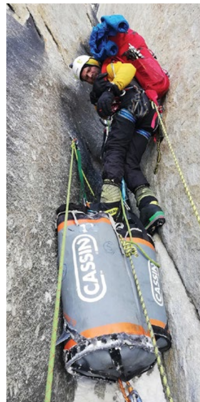
Lekkie holowanie. Podejście z workiem z osobistymi rzeczami, a następnie holowanie reszty sprzętu metodą przeciwwagi. Fot. Marcin Tomaszewski
