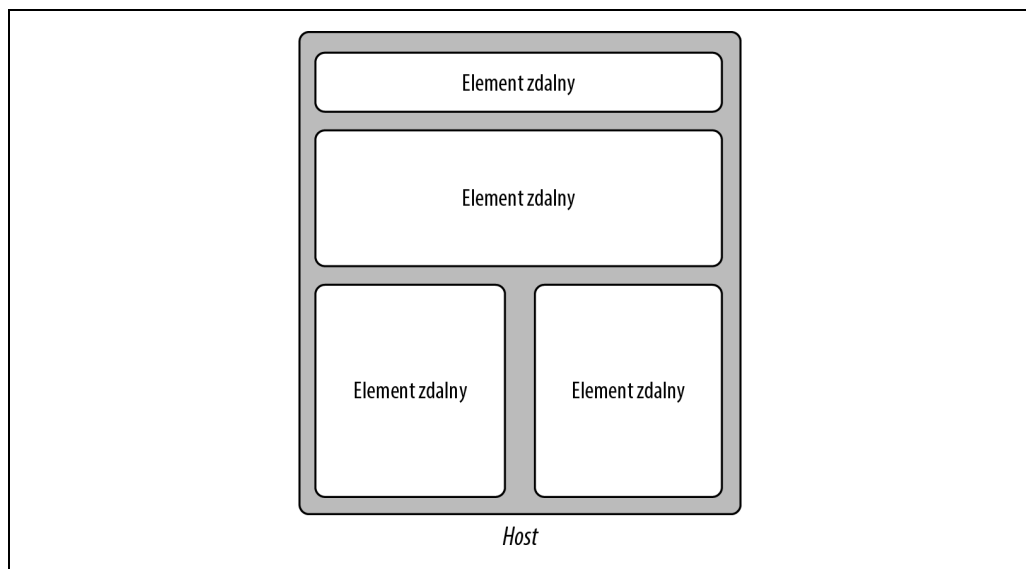
Rysunek 5.2. Wtyczka Module Federation składa się z dwóch kluczowych elementów: hosta, który ma za zadanie wgrywać paczki JavaScript w czasie działania aplikacji, oraz elementu zdalnego, który jest odpowiedzialny za paczki JavaScript, takie jak współdzielone biblioteki, mikrofrontendy, a nawet komponenty
