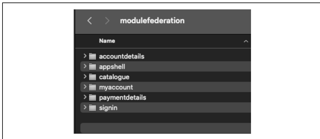
Rysunek 5.3. Struktura folderów projektu wewnętrznej aplikacji sklepu z drobiazгами
