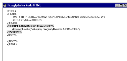
Rysunek 5.10. Poprzednia metoda deklaracji typu zastosowanego języka skryptowego
