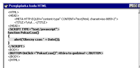
Rysunek 5.20. Przykładowy skrypt obrazujący wykorzystanie zdarzeń
