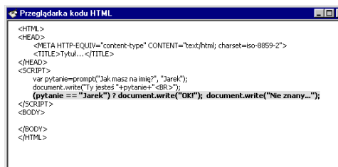
Rysunek 5.35. Uproszczona wersja instrukcji warunkowej if... else
