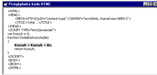
Rysunek 5.25. Przykłady operatorów w JavaScript, pierwszy jest operatorem przypisania, drugi operatorem matematycznym
