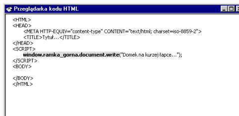
Rysunek 5.46. Przykład dziedziczenia obiektów. Aby wypisać tekst w ramce o nazwie „ramka_gorna” (zdefiniowanej gdzieś indziej) należy najpierw odwołać się do obiektu nadrzędnego window , następnie do podrzędnego mu obiektu ramki , dalej do podrzędnego tej ramce obiektu document i dopiero ostatecznie wywołać jej metodę write . Każdy kolejny poziom dziedziczenia został oddzielony kropką.
