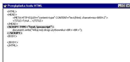
Rysunek 5.11. Metoda deklaracji wprowadzona w HTML 4.0
