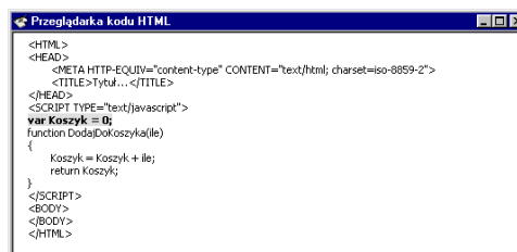
Rysunek 5.26. Nawet zwykłe zadeklarowanie zmiennej z jednoczesnym określeniem jej typu i nadaniem początkowej wartości, wiąże się z wykorzystaniem operatora przypisania
