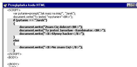
Rysunek 5.33. Przykład skryptu wykorzystującego instrukcję warunkową if ... else
