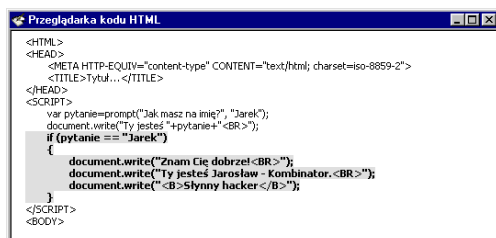
Rysunek 5.29. Fragment skryptu zawierającego instrukcję warunkową
