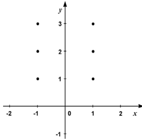
Rysunek 1.2.2. Interpretacja geometryczna zbioru \{-1, 1\} \times \{1, 2, 3\}
