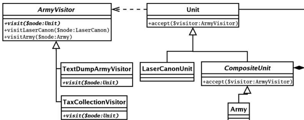
Rysunek 11.7. Wzorec Visitor
