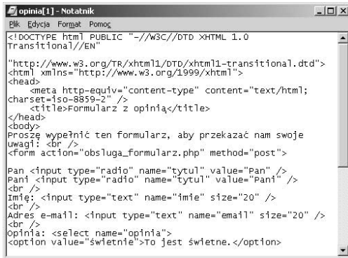
Rysunek 3.7. Przejrzyj źródło strony HTML, aby sprawdzić jej poprawność
