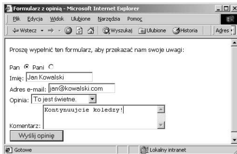
Rysunek 3.8. Wszystko, co użytkownik wpisze do formularza HTML, powinno być wyświetlone w przeglądarce WWW przez skrypt obsługi formularz.php (rysunek 3.9)
