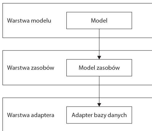
Rysunek 3.1. Schemat struktury modeli Magento
