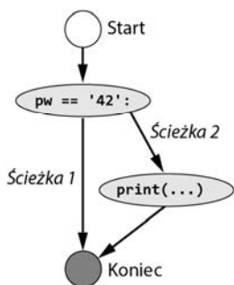
Rysunek 1.5. Złożoność cyklomatyczna dwóch programów Pythona
