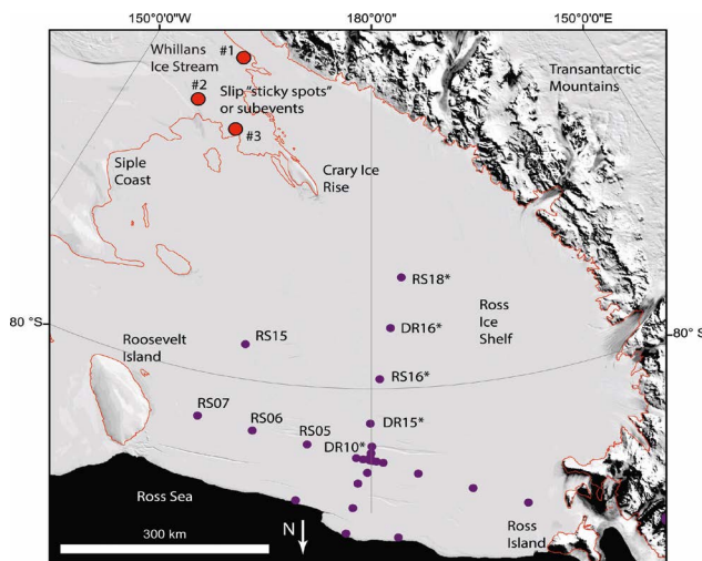
Lodowiec Szelfowy Rossa. Fioletowe punkty – lokalizacja sejsmometrów rejestrujących jego drżenia, czerwone – usytuowanie aparatury mierzącej ruch lodu.
