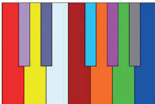
Ilustracja 2. Klawiatura Skriabina
