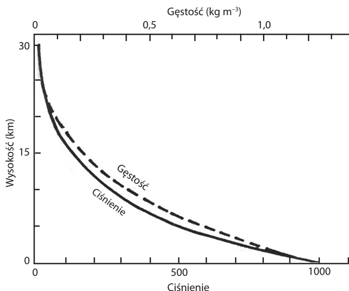
Rys. 1.1. Zmiany ciśnienia [hPa] i gęstości powietrza [kg/m³] w 30-kilometrowej warstwie atmosfery nad powierzchnią Ziemi
