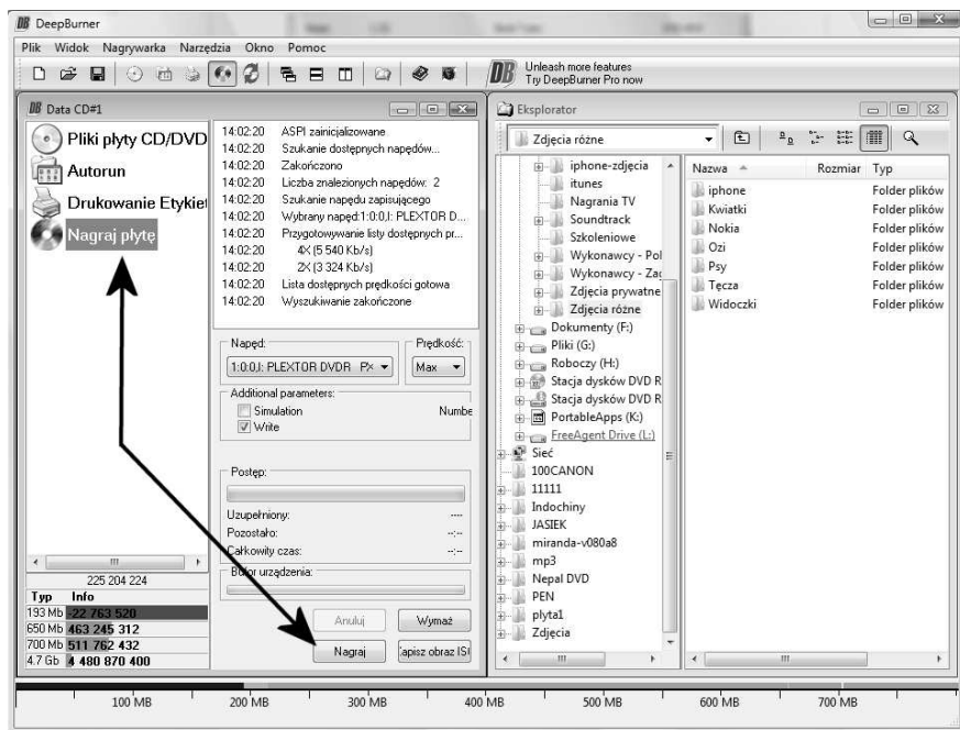
Rysunek 4.11. Przygotowanie płyty multisesyjnej za pomocą programu DeepBurner — etap czwarty
